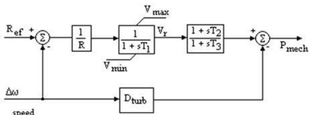
Fig. 4 Modelo Matemático de Regulador de Velocidade.
