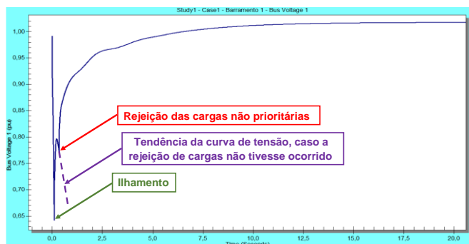
Fig. 8 – Tensão na Barra 1.
