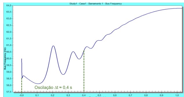
Fig. 6 – Frequência na Barra 1.
