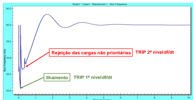
Fig. 9 – Frequência na Barra 1.
