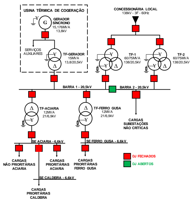
Fig. 1 Diagrama Unifilar Simplificado.
